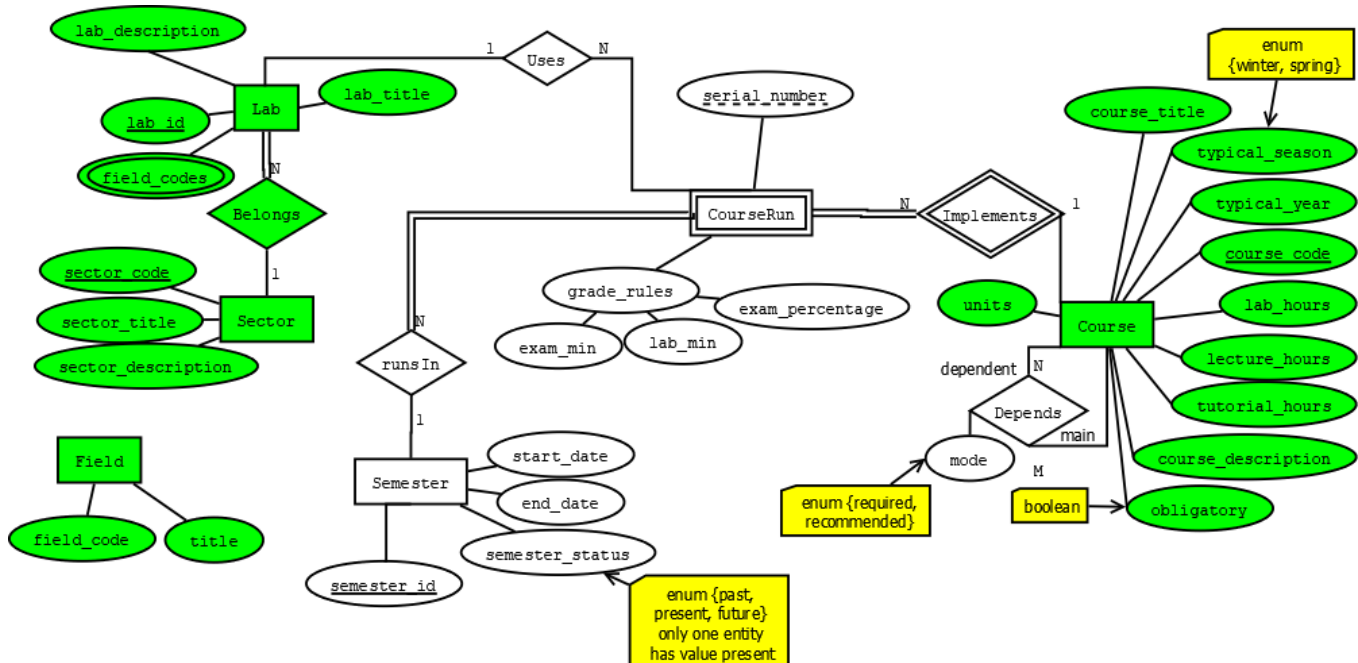
Διάγραμμα ER
